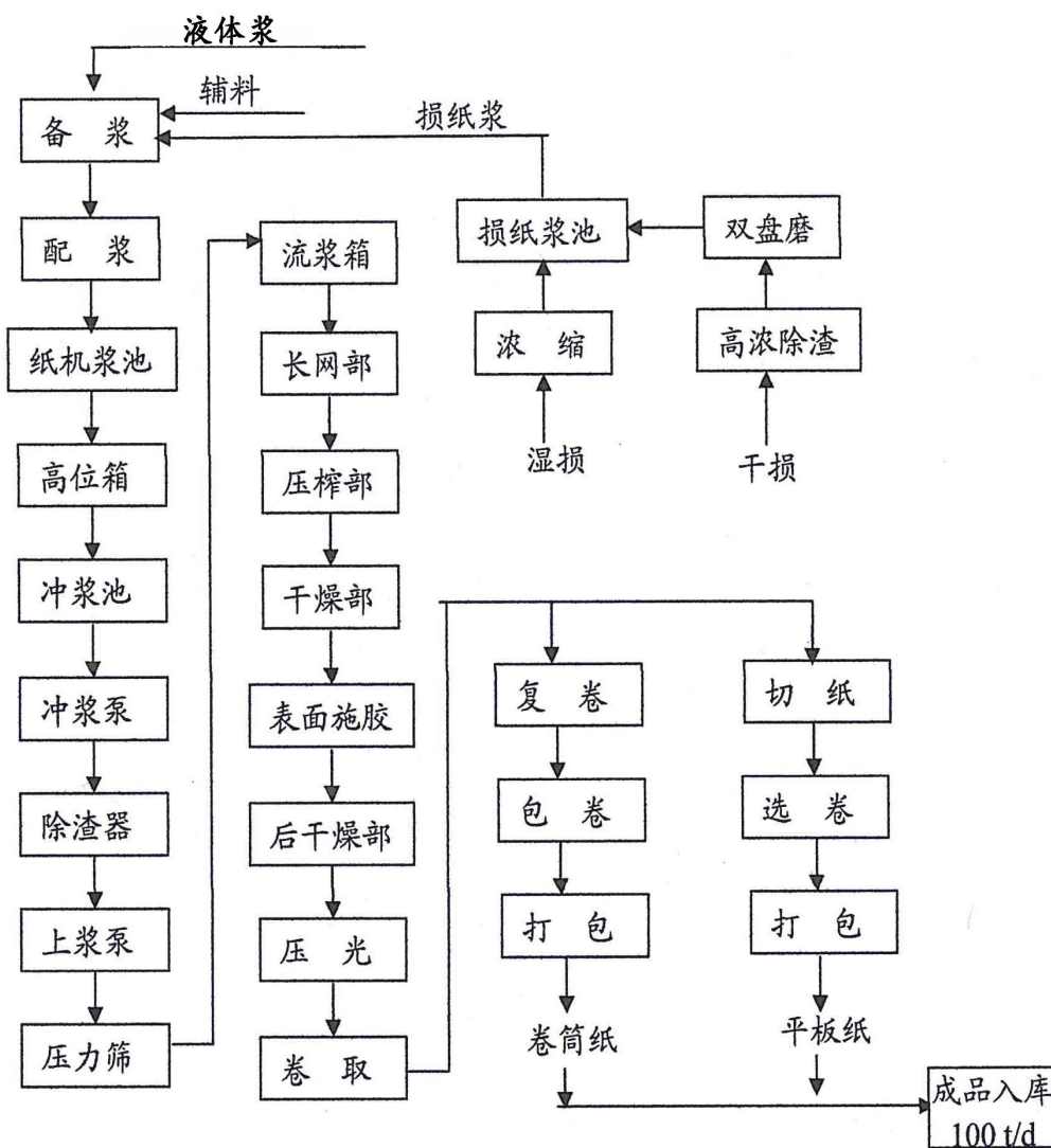
图 3-2 造纸工艺流程图
